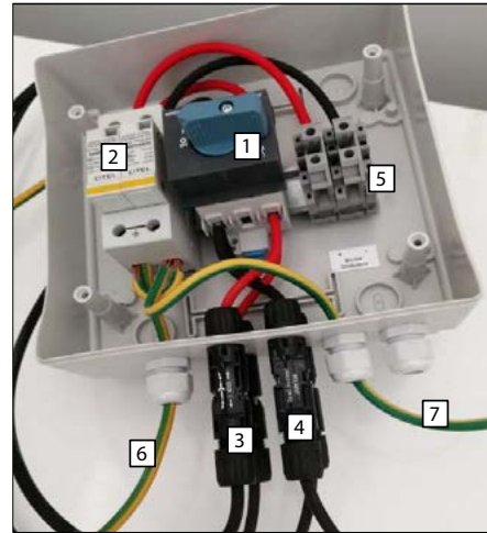
Coffret de protection PV
